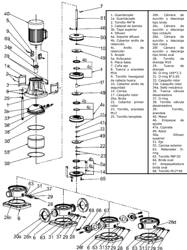
VMS(S)8,12,16,20 - TIPO A. INOX Figura 1 C
